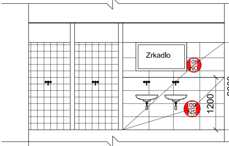
Pohľad
